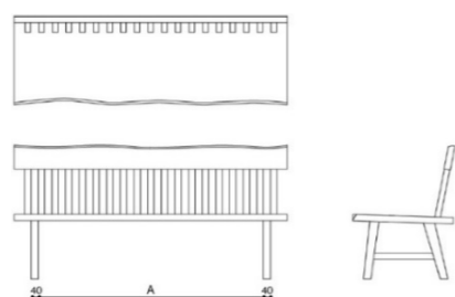
S-T1135 NOIL W1350×D約560×H約830×SH400
