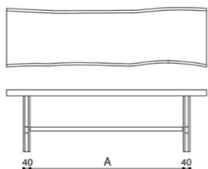
S-T3015 NOIL W1500×D約380×H400
